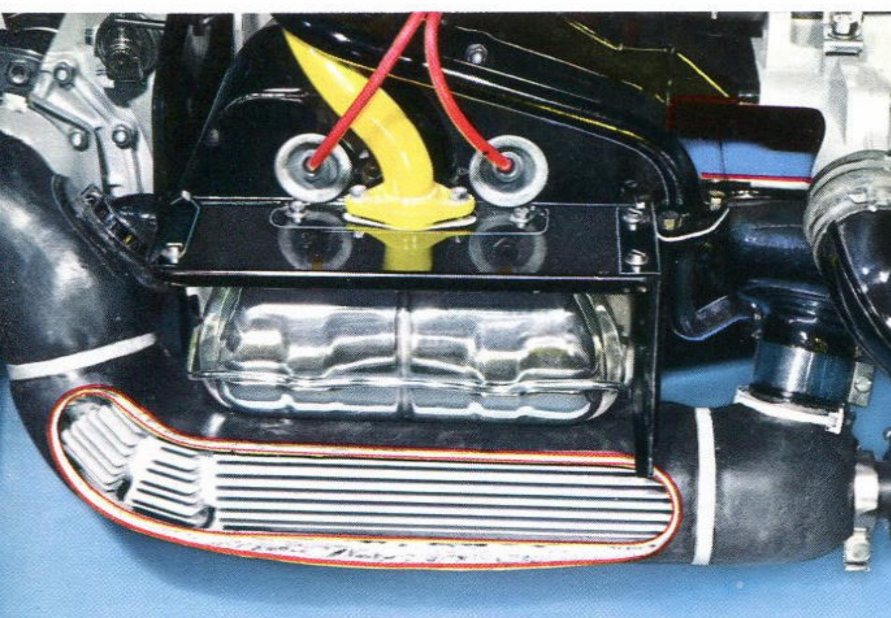
Här ett tvärsnitt av den ena av de båda värmeväxlarna, som är en del av den kompletta friskluftvärmeanläggningen, vilken är standard på VW 1500.
