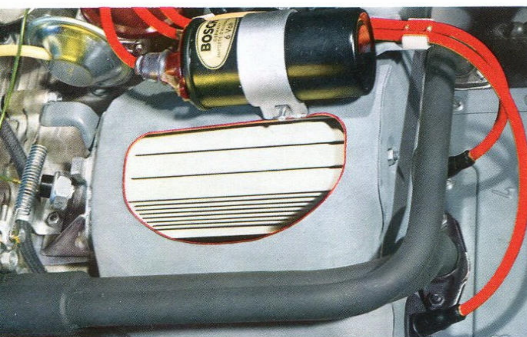
Den automatiskt reglerade oljekylaren är en av anledningarna till VW 1500-motorns enastående slitstyrka. Oljemängd: endast 2,5 liter. Oljebyte endast var 500:e mil.
